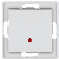
6027.x Sklopka naizmjenična sa indikacijom 10AX/250V~ Two-way switch with indication 10AX/250V~ • Indikacija svetli kada je strujno kolo otvoreno • Indication is on when the circuit is open
