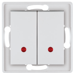
6026.x Sklopka serijska sa indikacijom 10AX/250V~ Serial switch with indication 10AX/250V~ • Indikacija svetli kada je sklopka isključena • Indication is on when the switch is off
