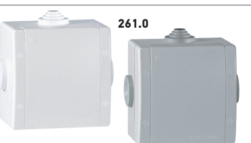
261.0 261.1 Kutija razvodna sa 3 uvođa za na zid 80x80 500V IP54 Wall mounted junction box with 3 cable glands 80x80 500V IP54
