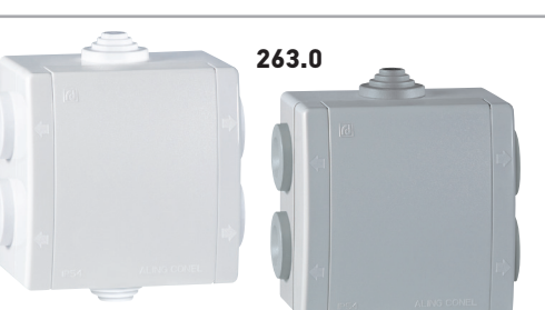
263.0 263.1 Kutija razvodna sa 6 uvođa za na zid 80x80 500V IP54 Wall mounted junction box with 6 cable glands 80x80 500V IP54
