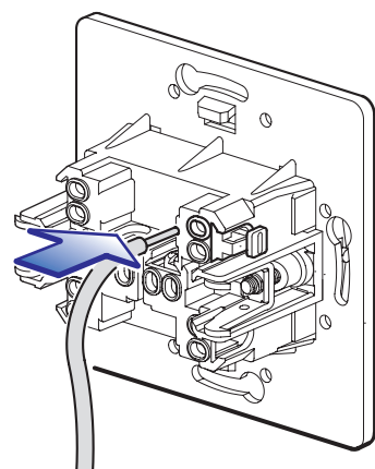
BEZVIJČANA MONTAŽA SCREWLESS INSTALLATION
